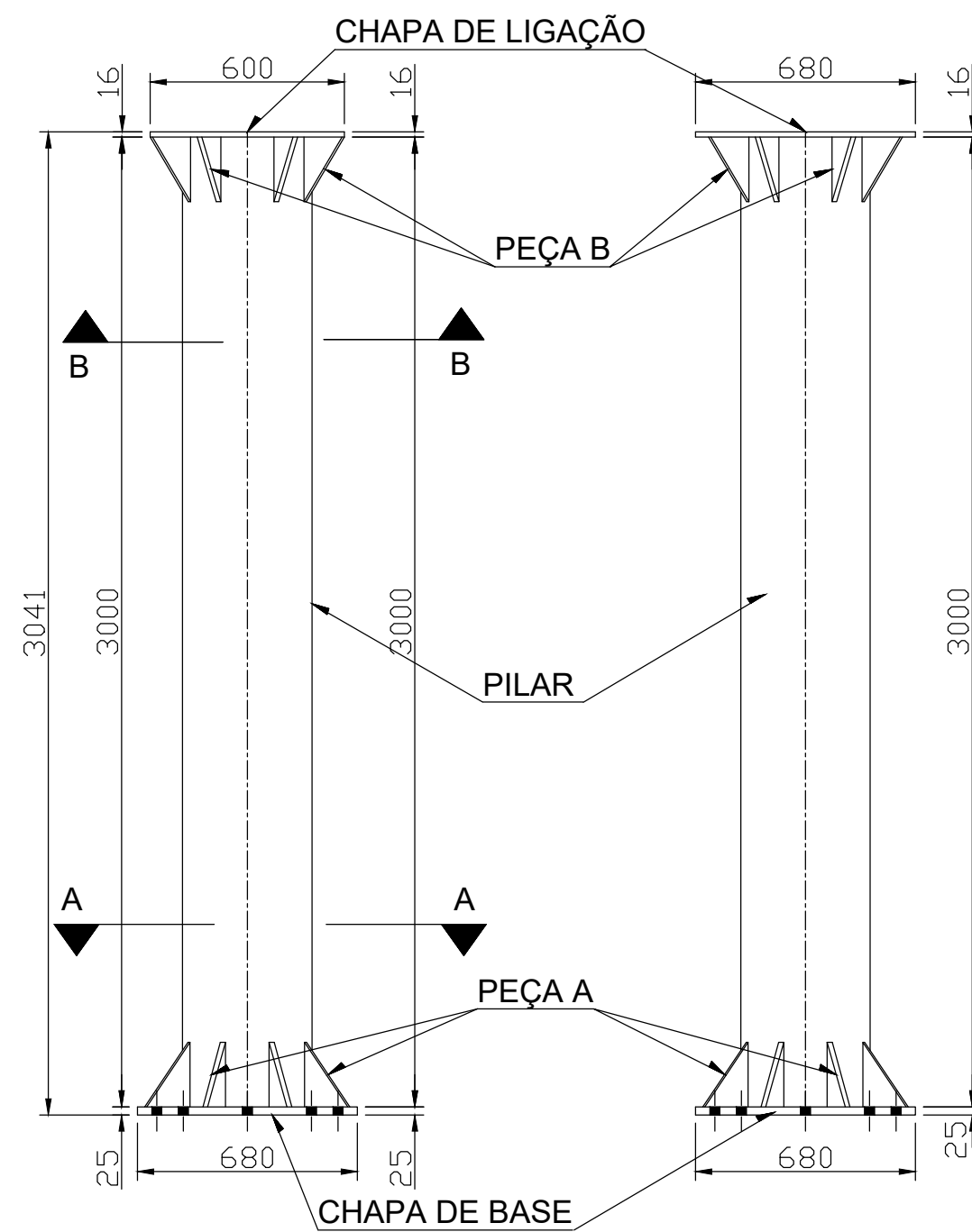
PILAR VISTA DA FRENTE QUANTIDADE: 01 PÇ
