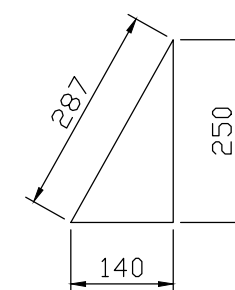
PEÇA A CHAPA # 3/8" QUANTIDADE : 16 PÇS
