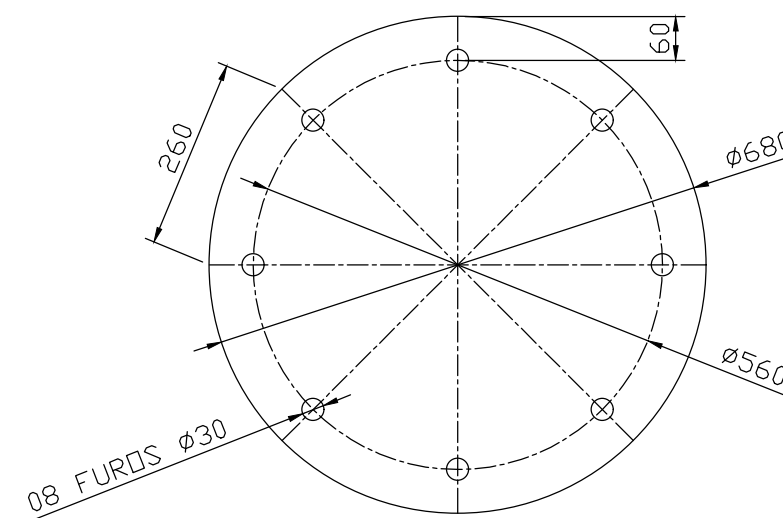
CHAPA DE BASE CHAPA # 1" QUANTIDADE: 02 PÇS
