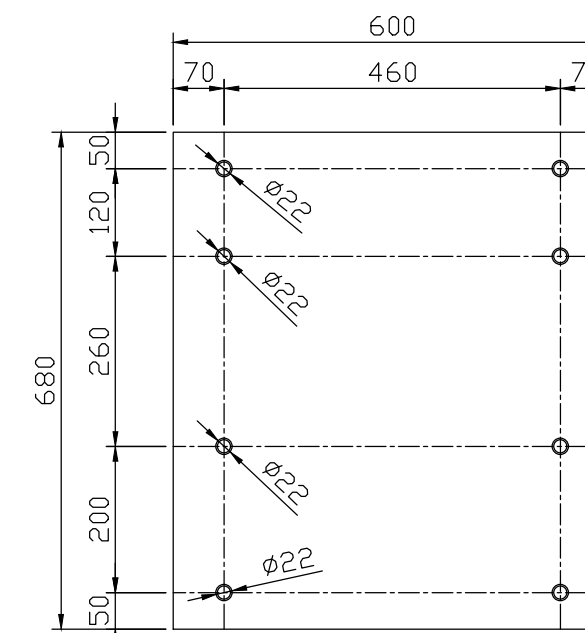
CHAPA DE LIGAÇÃO CHAPA # 5/8" QUANTIDADE: 04 PÇS
