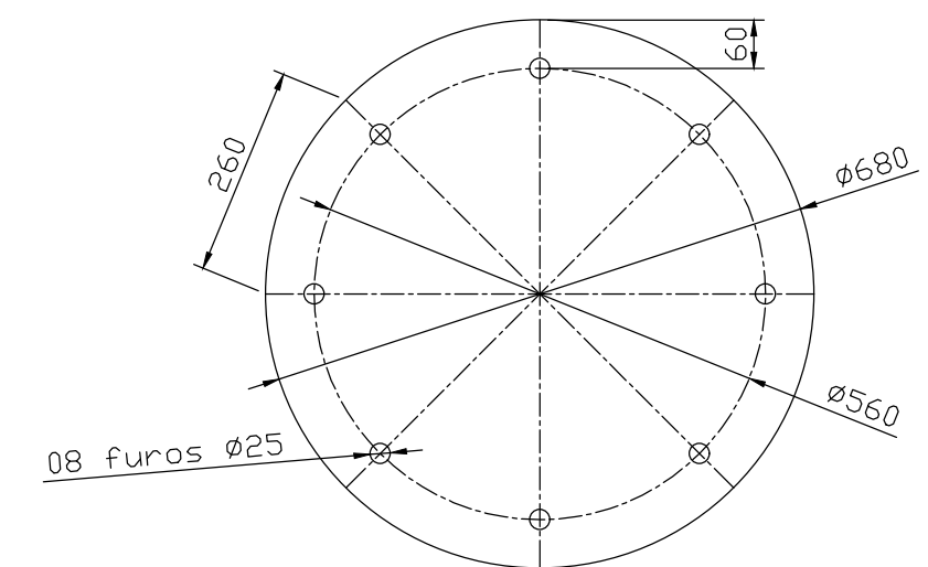
CHAPA GABARITO CHAPA # 14" QUANTIDADE: 02 PÇS
