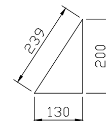
PEÇA B CHAPA # 3/8" QUANTIDADE : 16 PÇS
